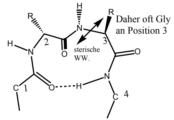
\beta -Turn (Typ 2)
